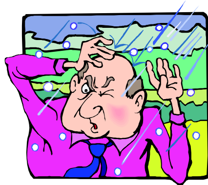
grêle
