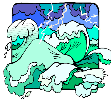
tempête
