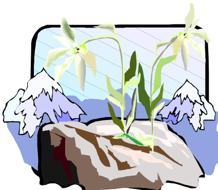
Première floraison
