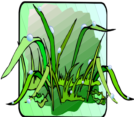
Rosée
