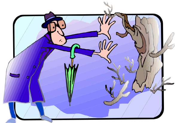
verglas
