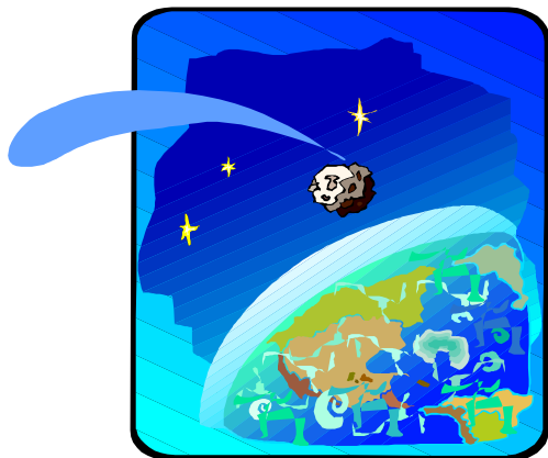
Météorite
