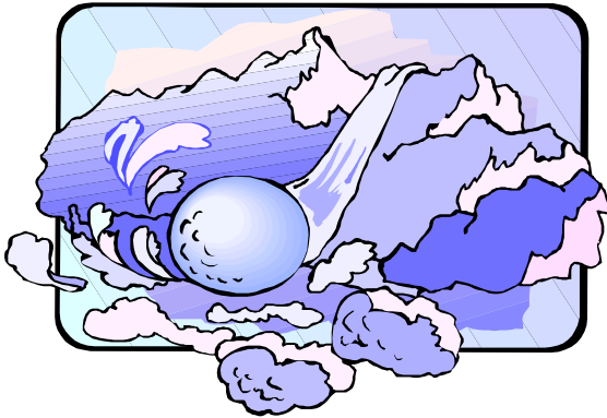
Avalanche
